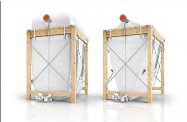
Abb. 12: Ausdehnung eines luftdurchlässigen Gewebesilos im gefüllten und leeren Zustand
