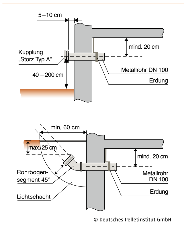
Abb. 21: Anforderungen an die Zugänglichkeit der Befüllstutzen im Freien und im Lichtschacht
